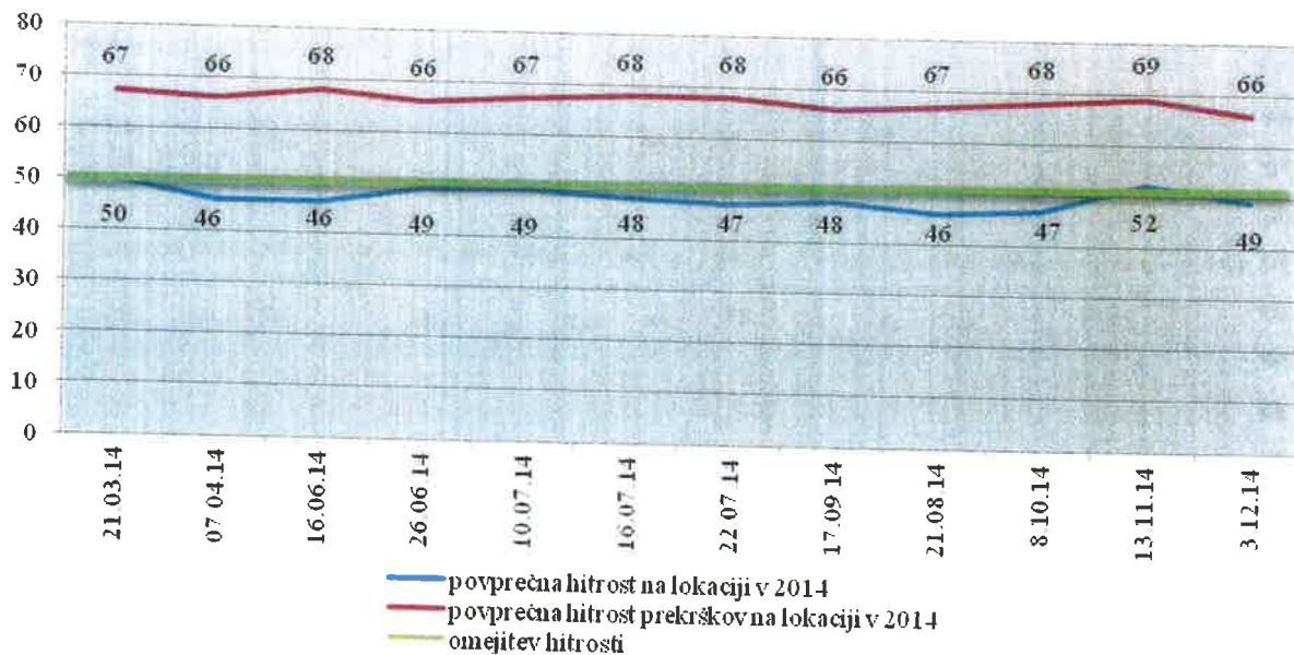
Slika 22: Razmerje med povprečnimi hitrostmi vseh izmerjenih vozil in povprečnimi hitrostmi prehitrih vozil na Dunajski cesti v Prevojah v Lukovici.
