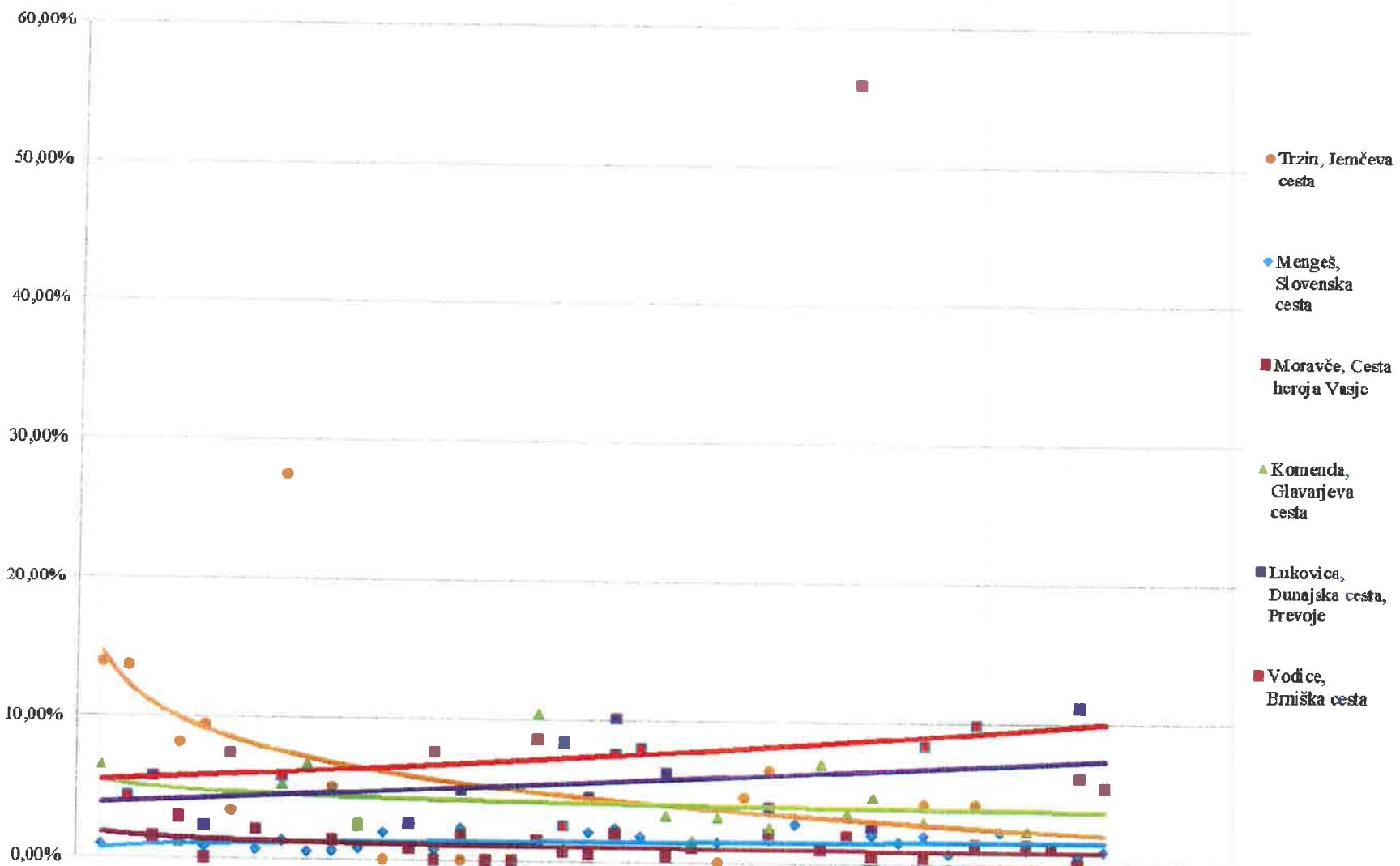
Slika 29. Delež kršitev na izbranih lokacijah glede na vsa izmerjena vozila, po posameznih meritvah, tekom leta.
