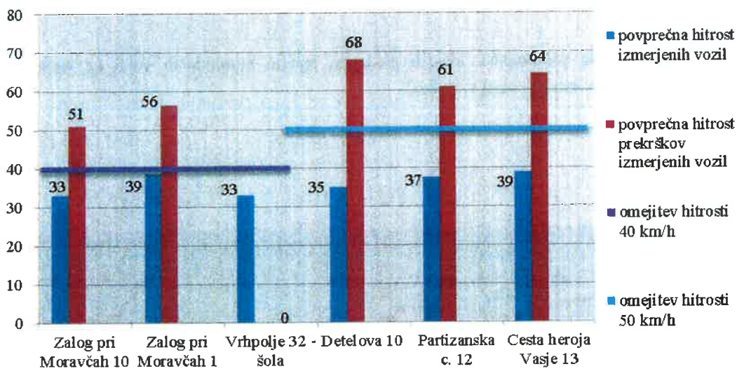
Slika 15: Razmerje med povprečnimi hitrostmi vseh izmerjenih vozil in povprečnimi hitrostmi prehitrih vozil na posameznih lokacijah v Občini Mengeš.
