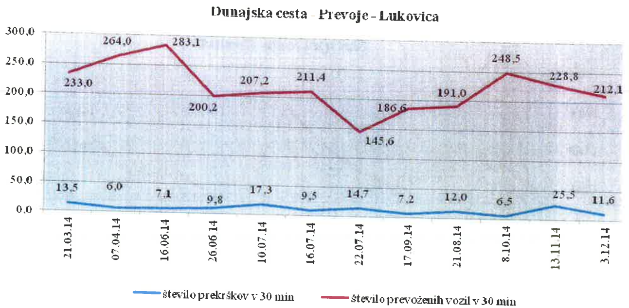
Slika 21: Razmerje med številom prekoračitev hitrosti glede na število mimoidočih vozil na enoto časa v posameznih meritvah na Dunajski cesti v Prevojah v Lukovici.
